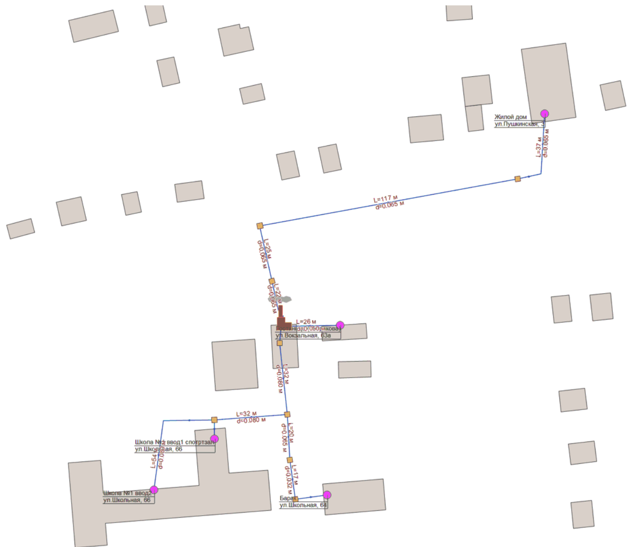
Рисунок 2.2.8 Схема тепловых сетей. Котельная №9
