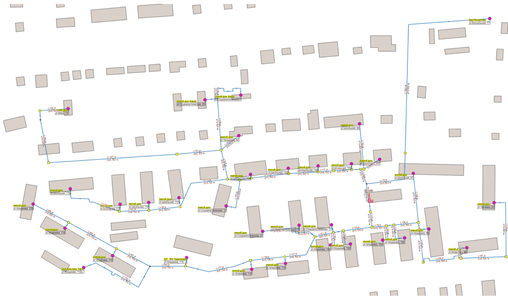
Рисунок 2.2.1 Схема тепловых сетей. Котельная №1
