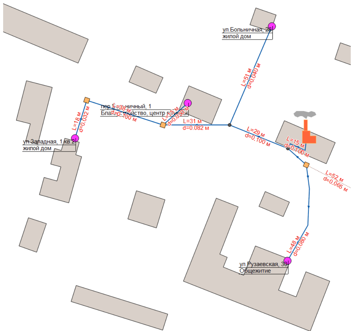
Рисунок 2.2.10 Схема тепловых сетей. Котельная №11
