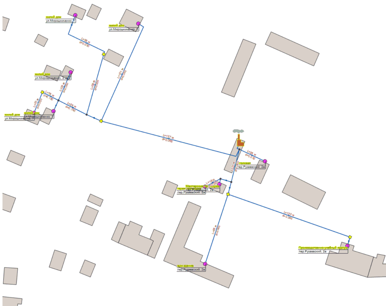
Рисунок 2.2.6 Схема тепловых сетей. Котельная №7
